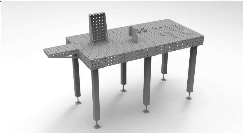
Макет сварочно-сборочный стол 2000x1000 6мм
